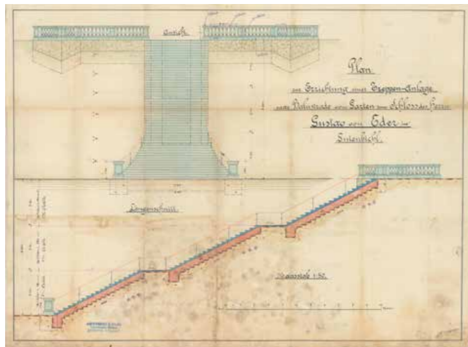
Načrt stopnišča pred dvorcem Marof, hrani Knjižnica Velenje
