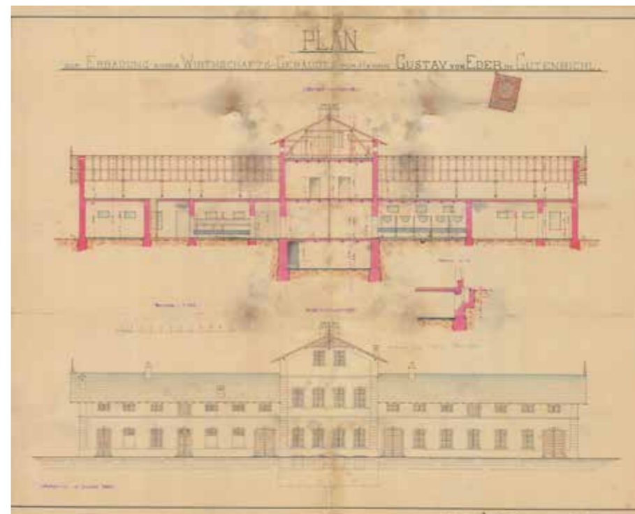
Načrt gospodarskega poslopja dvorca Marof, hrani Knjižnica Velenje
